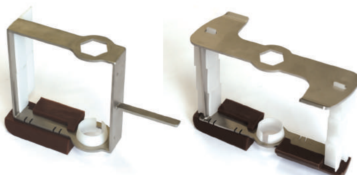
Bras de mélange livrés avec le RT51 - R52 MAX
