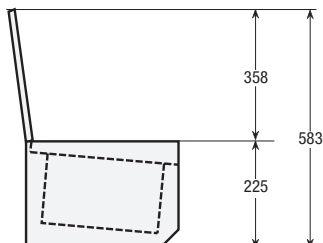
Vue en coupe de la vitrinette avec le couvercle inox
