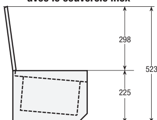
Vue en coupe de la vitrinette avec le couvercle inox
