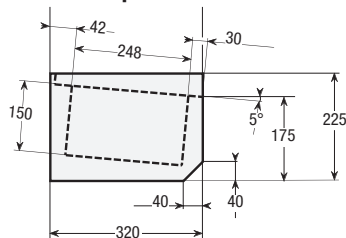
Vue en coupe de la vitrinette avec le couvercle inox
