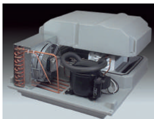
Unité frigorifique monobloc BREVETÉE
