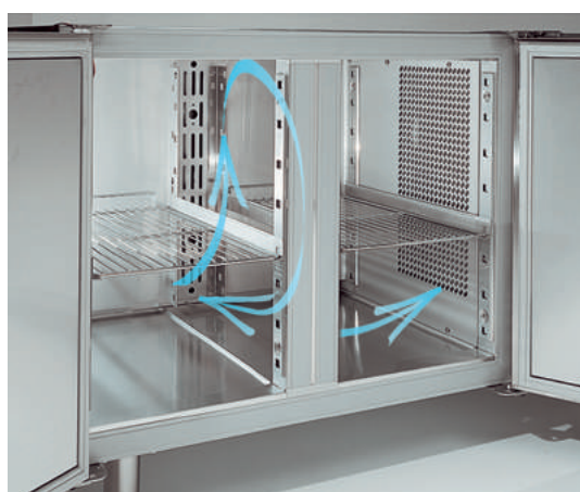
Système de ventilation
